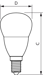
CorePro lustre ND 5-40W E14 827 P45 FR
