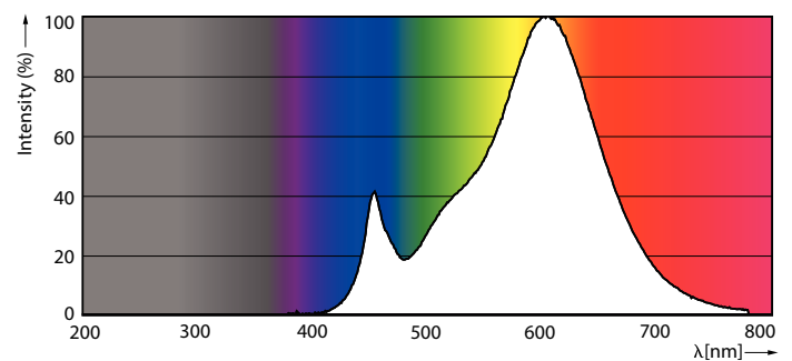
LEDlustrer CorePro 7W P48 E27 827 FR-POC
