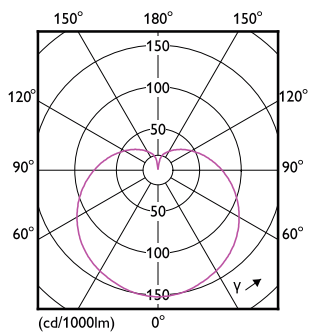
LEDlustrer CorePro P48 7W E27 827 FR-LDD
